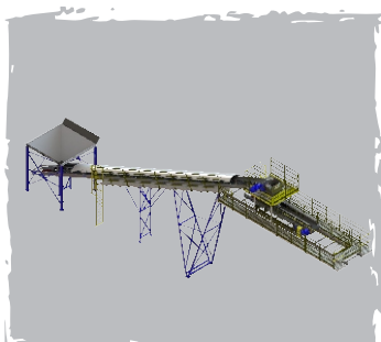
Sistema de alimentação de agregados com carro de translação para CDR-80
