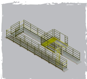
Plataforma superior para caixa de agregados da CDR-80
