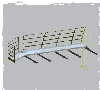
Passadiço para transportador
